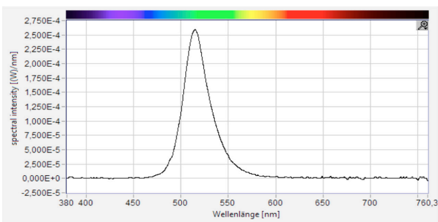
24 Vdc RGB+WW Flex 72 Grün
